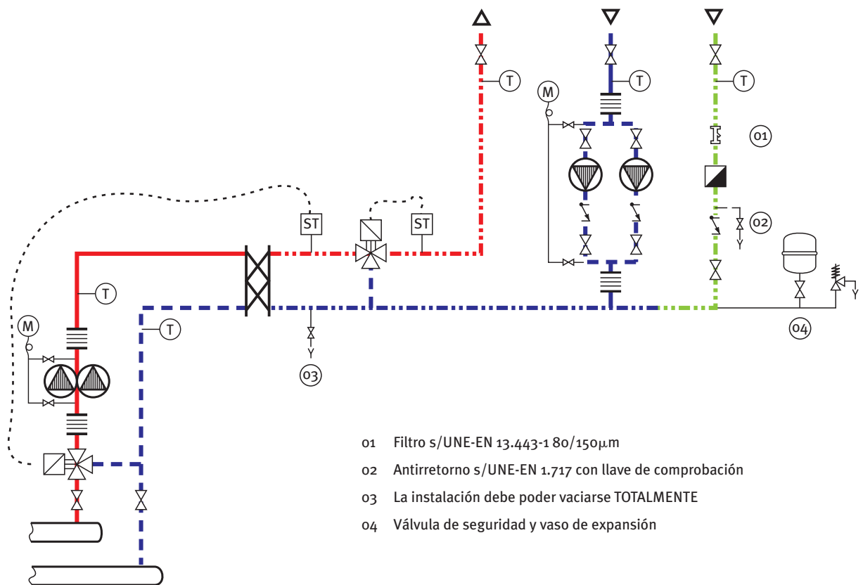
Fig. 04: Producción instantánea de ACS. Regulaciones en primario y secundario. Bombas dobles en primario y recirculación
