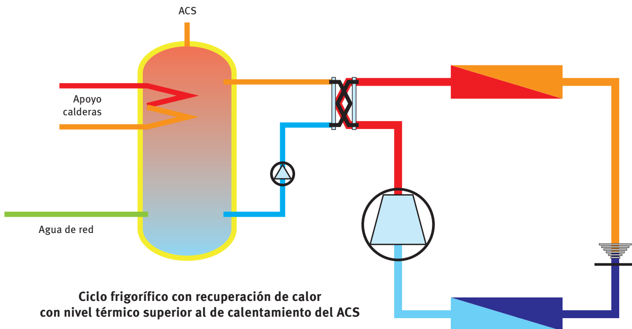
Fig. 23A: Aportación de la recuperación de calor al depósito de consumo; apoyo de calderas mediante interacumulador
