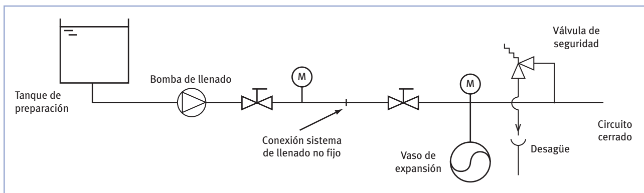
Figura 22: Esquema de llenado mediante depósito
